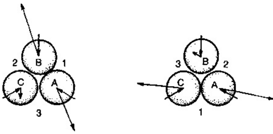
Şekil 5.8. Bir üçlü çarpışma. Sonuçtaki davranış, hangi parçacıkların önce bir araya geldiklerine bağlıdır ve bu nedenle sonuç sürekli biçimde girdiye bağlıdır.
