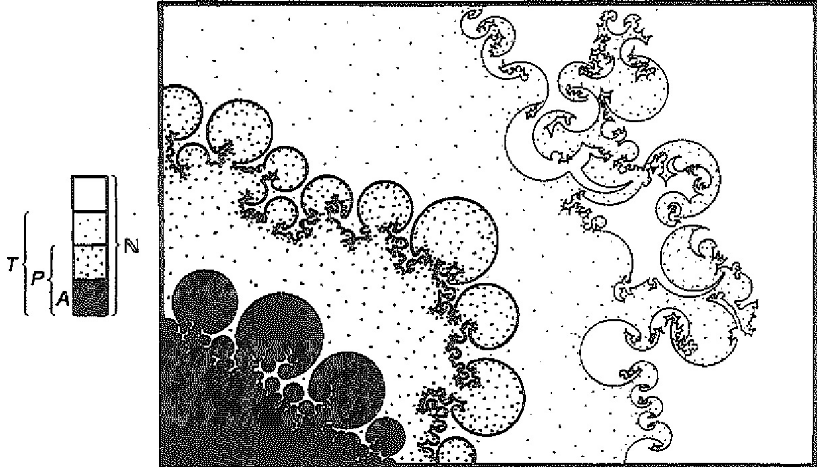
Şekil 4.3. Çeşitli önermeler kümelerinin son derece şematik tasarımı. Sistemde
