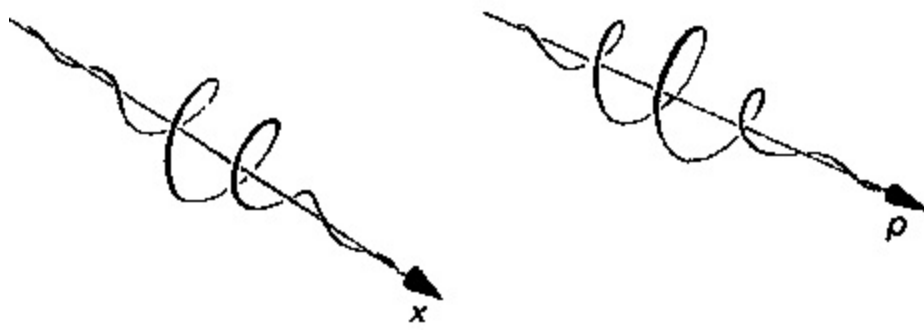
Şekil 6.14. Dalga paketleri. Bunlar hem konum uzayında hem de momentum uzayında yerelleşmiştir.
