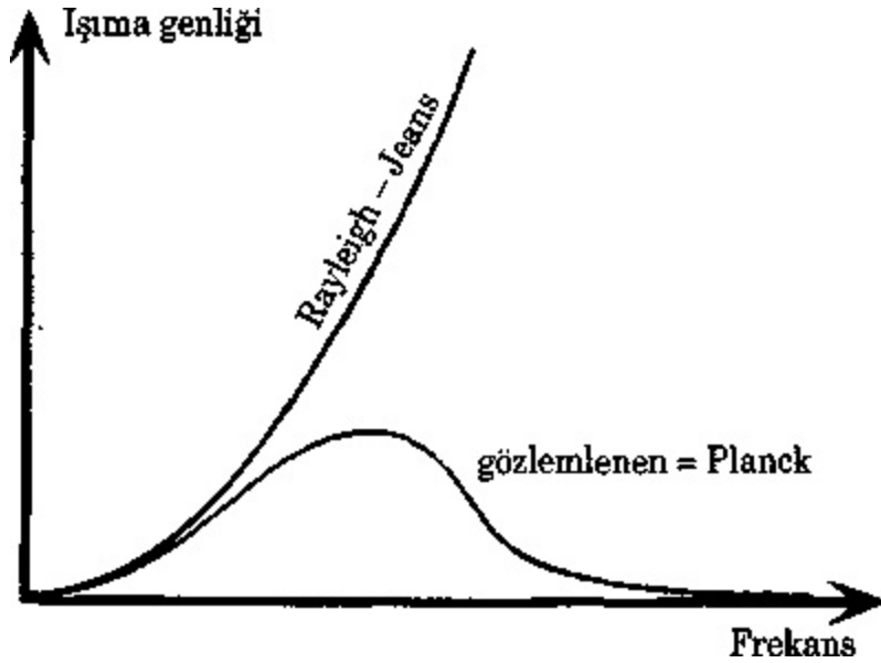
Şekil 6.2. Sıcak bir cismin ('siyah cisim') ışıma genliğinin klasik yöntemle (Rayleigh-Jeans) ve gözlemlenilen değerleri arasındaki farktan hareketle Planck, kuantum kuramının ilk aşamasını başlattı.
