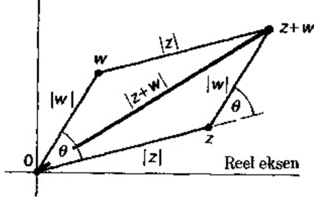
Şekil 6.9. İki genliğin toplamının mutlak değer karesi için 2|w||z|\cos\theta düzeltme terimini veren geometri
