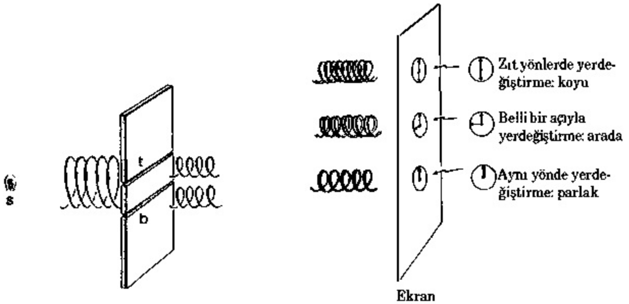
Şekil 6.13. İki yarık deneyinin foton momentum durumlarının sarmal tanımla analizi.
