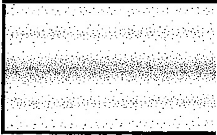
Şekil 6.5. Her iki yarık da açık olduğundaki genlik kesikli noktaların dalgali dağılımını gösterir.
