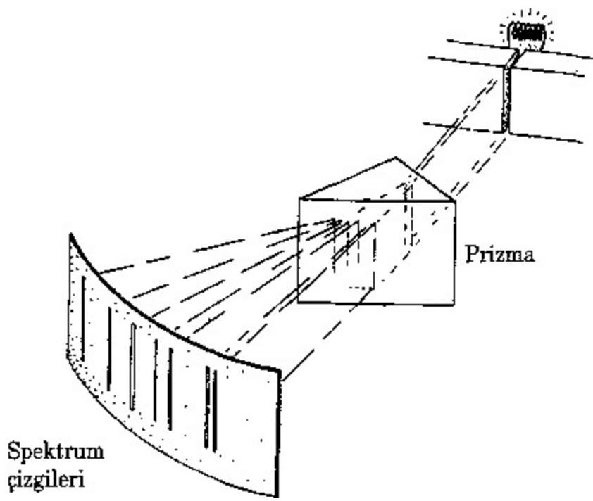
Şekil 6.1. Isıtılan bir maddedeki atomlar, özgül frekanslarda ışık yayarlar. Bu ışık, bir prizmadan geçirilerek, atomların özelliğini yansıtan spektrum çizgileri kümesi oluşturulur.
