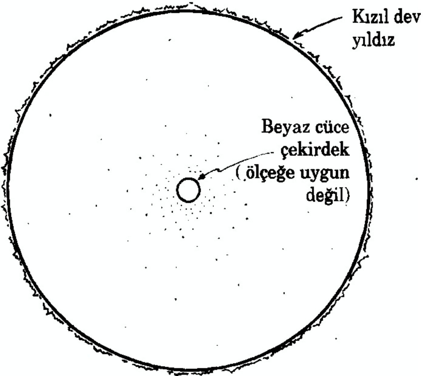
Şekil 7.12. Beyaz cüce çekirdekli bir kızıl dev.
