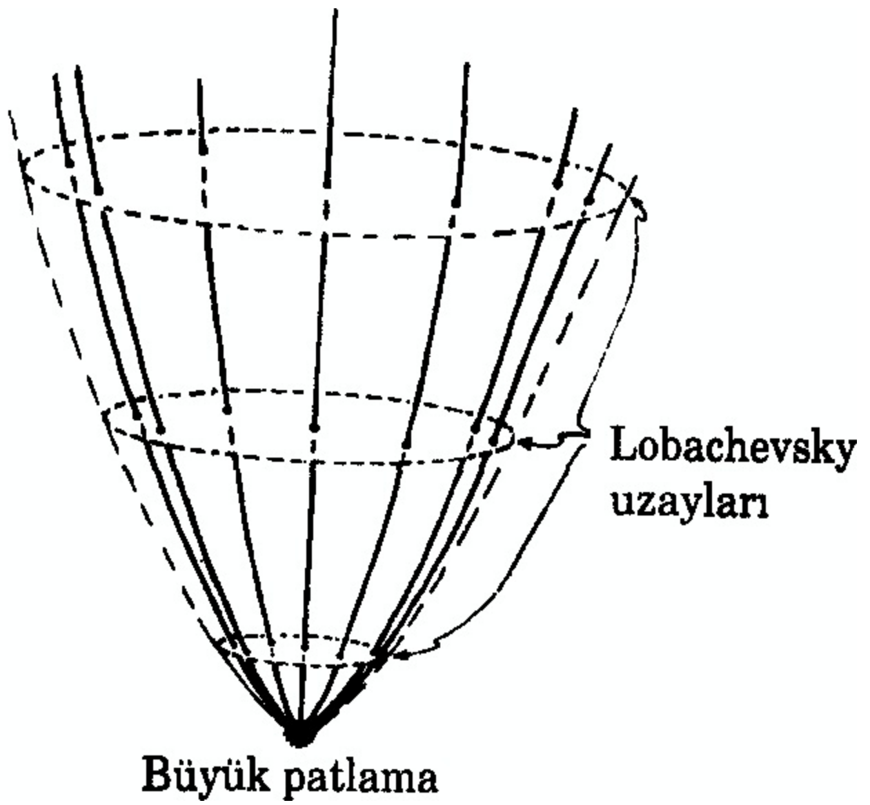
Şekil 7.10 Uzaysal kesitleri Lobachevsky uzayı olan bir genişleyen evrenin uzay-zaman şeması (sadece iki uzay boyutu gösterilmiştir).
