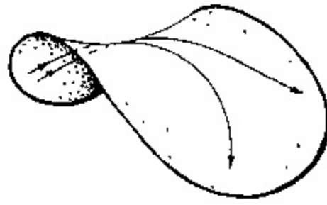
Eksi eğrilikli yüzey
