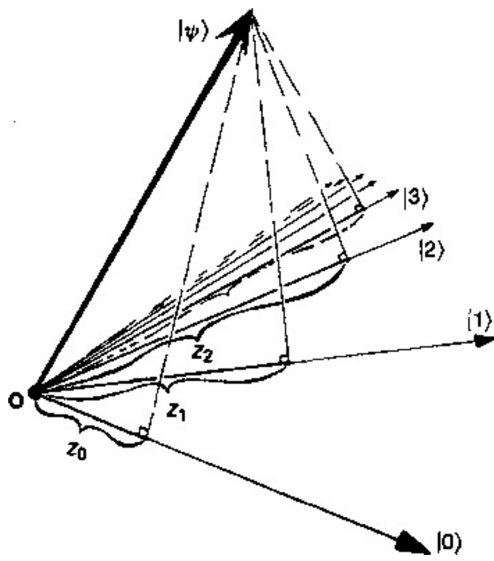
Şekil 6.22. |\psi\rangle durum vektörünü |0\rangle, |2\rangle, |2\rangle \dots |\psi\rangle durum vektörünün eksenleri üstüne düşey izdüşümlerinin boyları, öngörülen z_0, z_1, z_2 \dots genliklerini verir.
