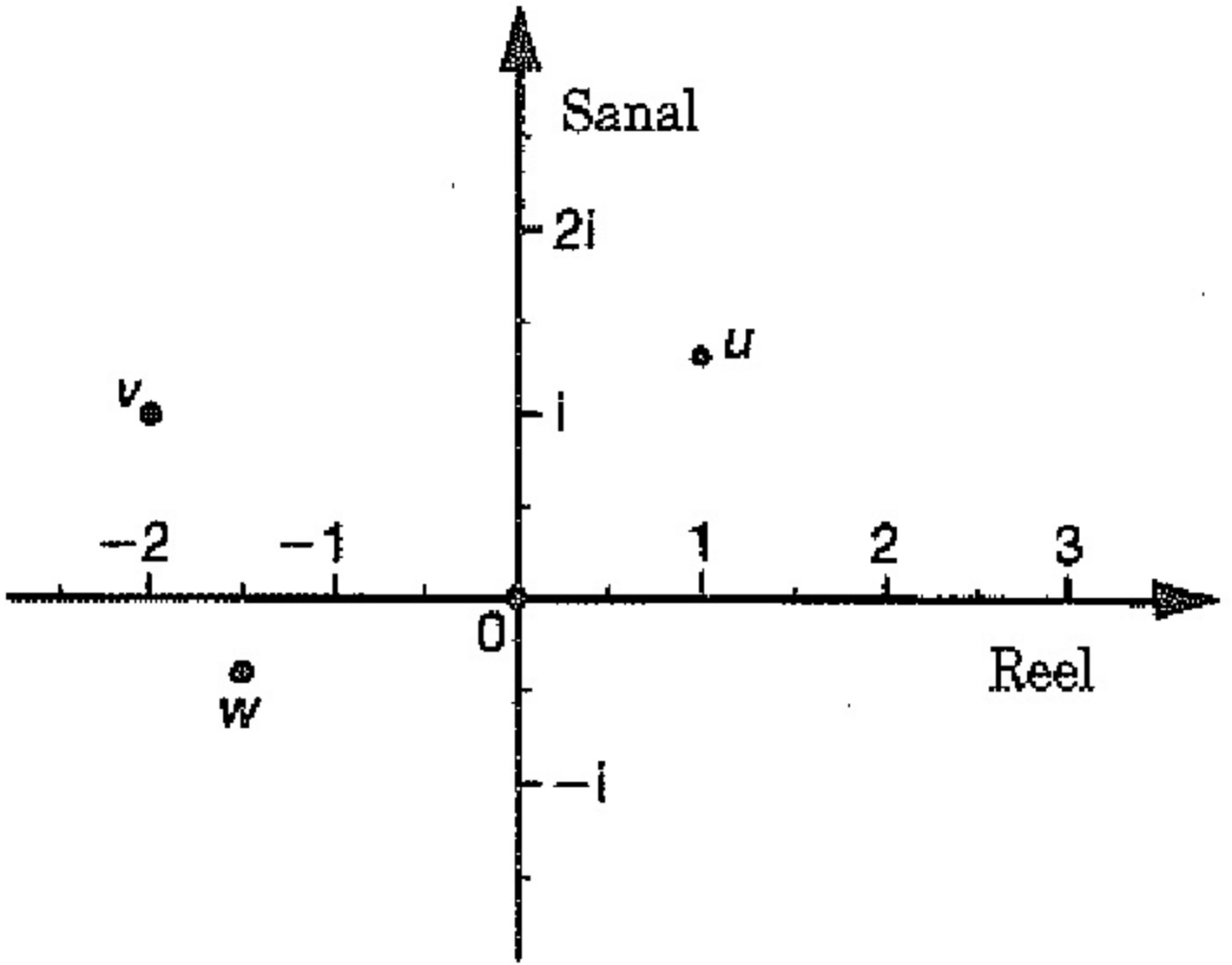
Şekil 3.9: u = 1 + i , v = -2 + i , ve w = -1.5 - i noktalarının Argand düzlemindeki yerleri.
