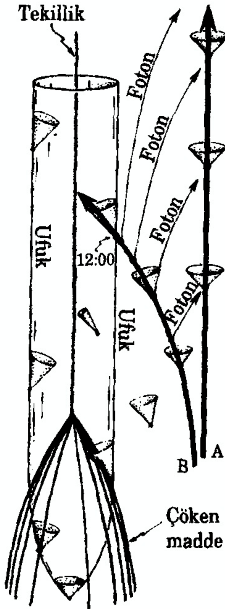
Şekil 7.13. Kara deliğe dönüşümü gösteren bir uzay-zaman şeması. Schwarzschild
