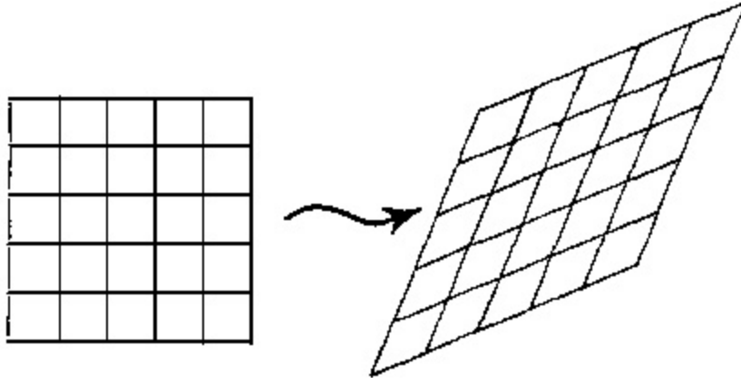
Şekil 5.20. İki uzay-zaman boyutunda bir Poincaré hareketi.
