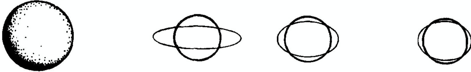
Şekil 7.15. Kütleçekim etkisi yaratan küresel bir cisimden kaynaklanan gelgit etkisi cisime yaklaştıkça, cismin merkezinden uzaklığın kübünün tersine orantılı olarak artar.
