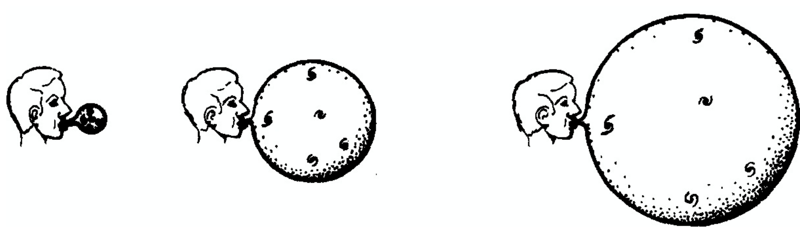
Şekil 7.8. Evrenin genişlemesi, şişirilmekte olan bir balonun yüzeyine benzetilebilir. Galaksiler birbirlerinden uzaklaşmaktadırlar.
