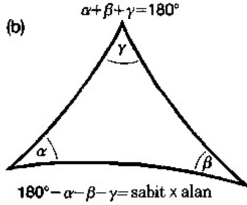
Şekil 5.1. (a) Eukleides uzayında bir üçgen, (b) Lobachevsky uzayında bir üçgen.
