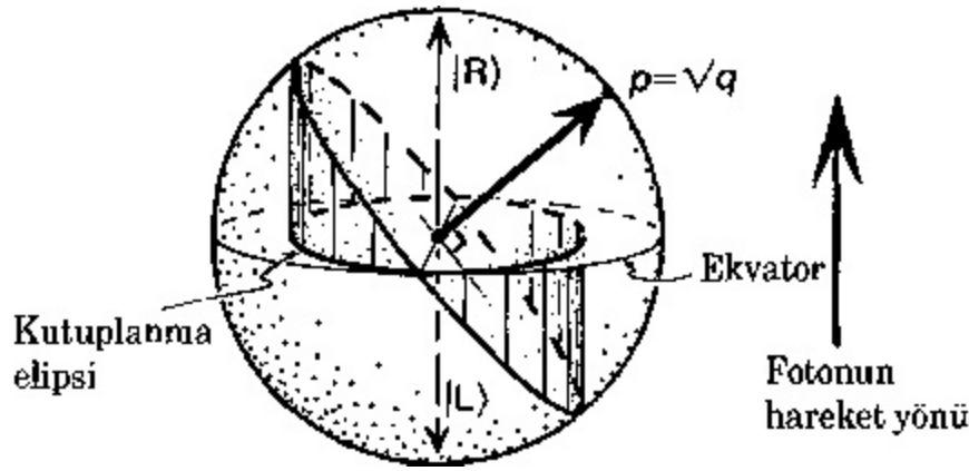
Şekil 6.28. \sqrt{q} 'nın Riemann küresi ile bir fotonun kutuplanma durumları tanımlanır.
