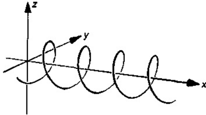
Şekil 6.11. Bir momentum durumunun, \psi eğrisi sarmal yapıdadır.
