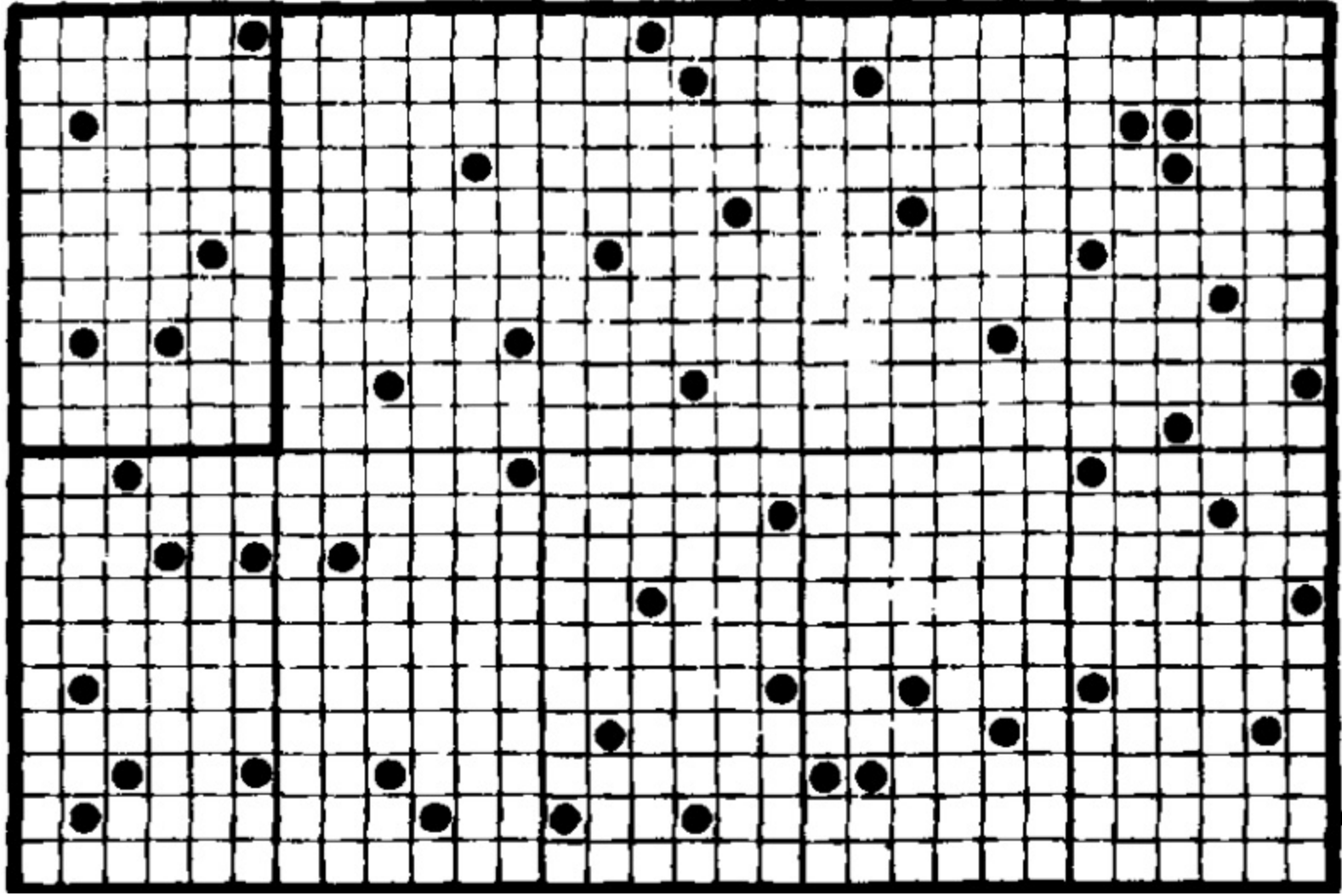
Şekil 7.4. Kutu içindeki gazla ilgili bir örnek: Belli bir sayıdaki minik toplar, daha fazla sayıda hücelere dağıtılmıştır. Kutucuklardan bazıları ‘özel’ olarak işaretlenmiştir. Bunlar sol üst köşede görülmektedir.
