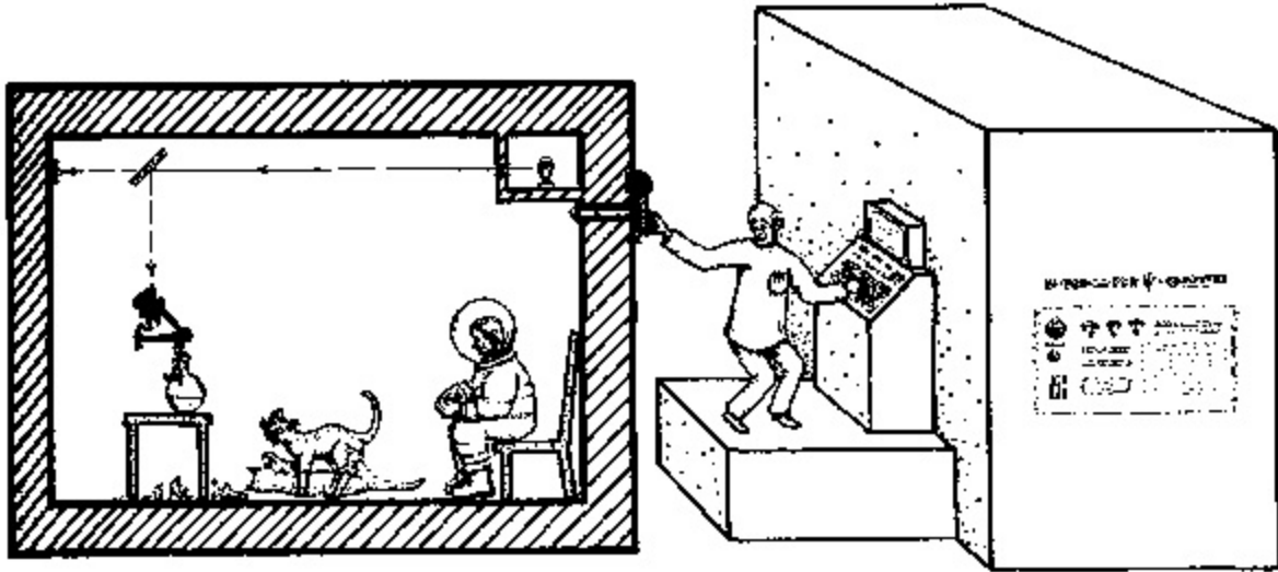
Şekil 6.33. Schrödinger'in kedisi-eklemeler yapılmış haliyle.
