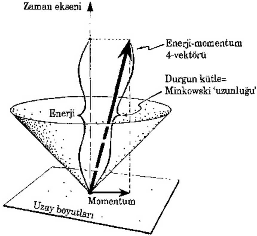
Şekil 5.35. Enerji-momentum 4-vektörü
